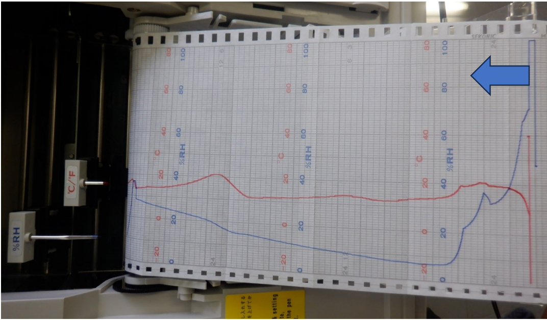
ST-50A温湿度計 温度(赤色)湿度(青色)推移 (2.5mm/h) 約3日稼働記録
